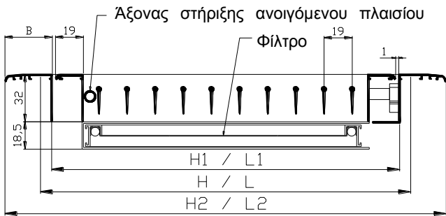
WS-101-A-F - ΤΟΜΕΣ
